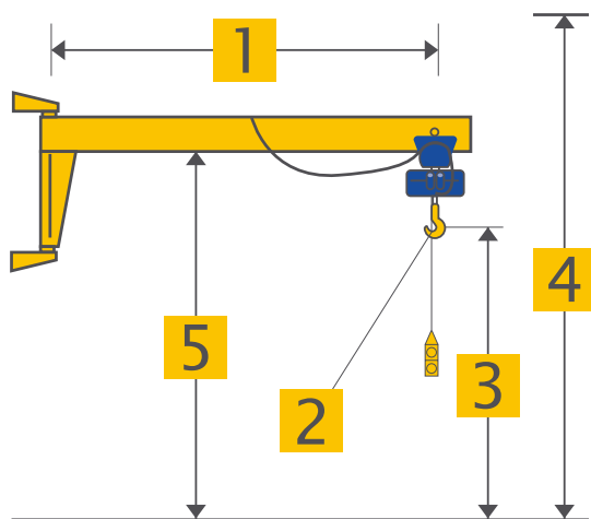
Настенный консольный кран
